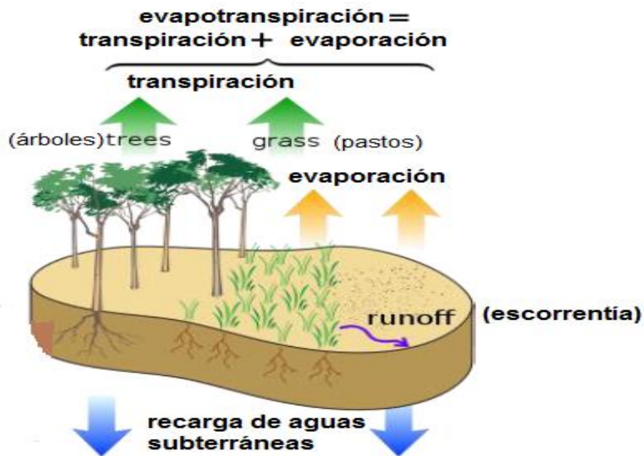
Figura 2. Evapotranspiración dividida en sus dos componentes y su relación con el área foliar por unidad de superficie del suelo. Fuente: USGS EROS/NCS CSC.
