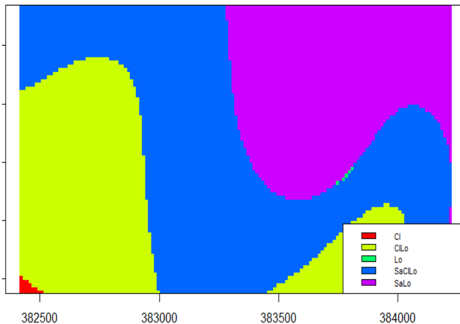
Figura 24. Suelos de la cuenca Challana, CI (Arcilla), CI Lo (Franco Arcilloso), Lo (Franco), SaCI Lo (Franco Arcilloso Arenoso), SaLo (Franco Arenoso)
