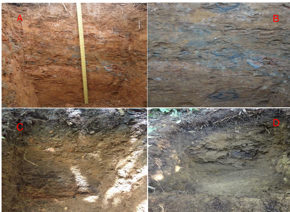
Figura 39. Perfil de suelos de algunos puntos de muestreos, A: suelo para pasto, B: suelo para purmas, C: suelo para bosques aproximadamente de 30 años, D: suelo para bosque de 20 años aproximadamente.
