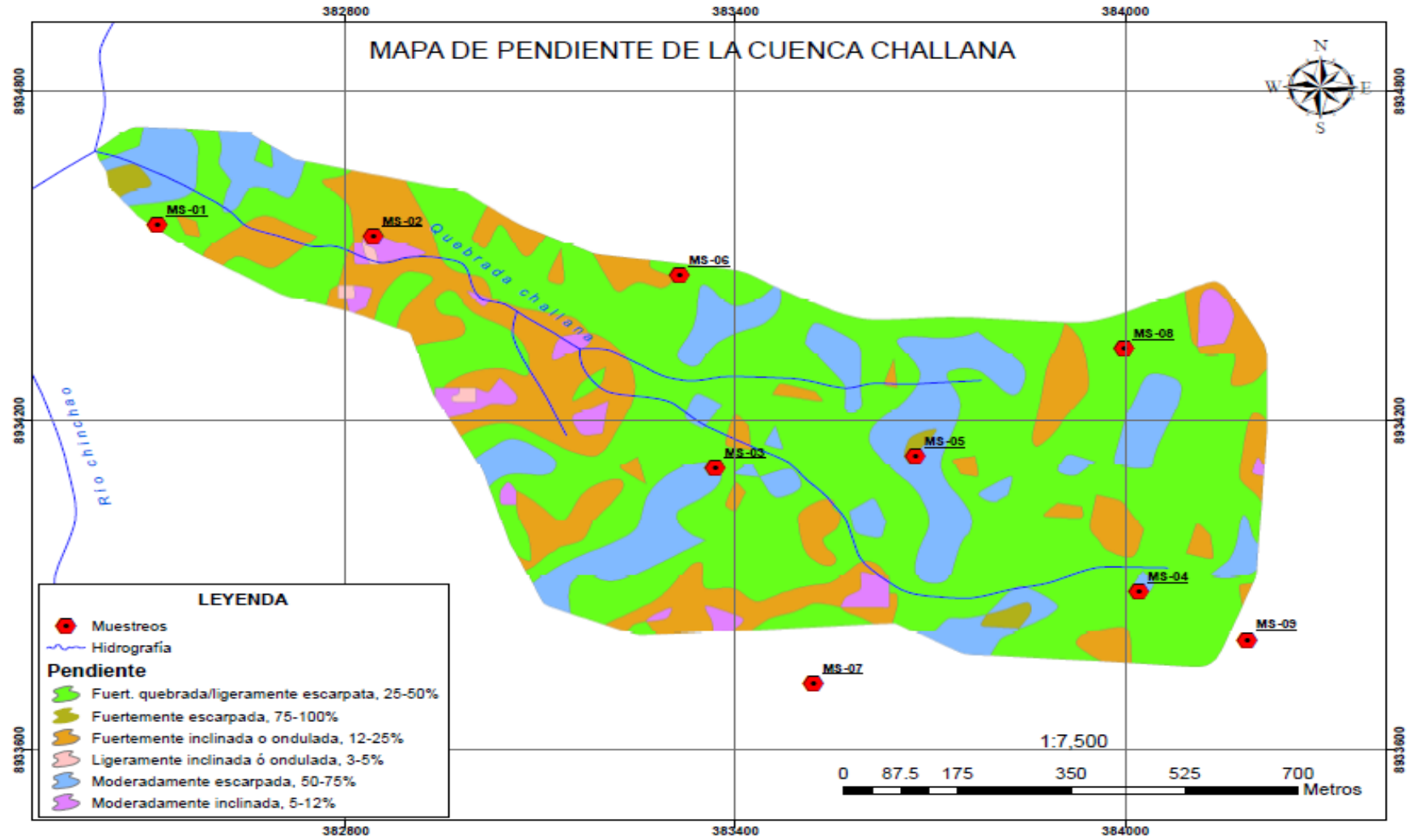
Figura 21. Mapa de pendiente de la cuenca Challana
