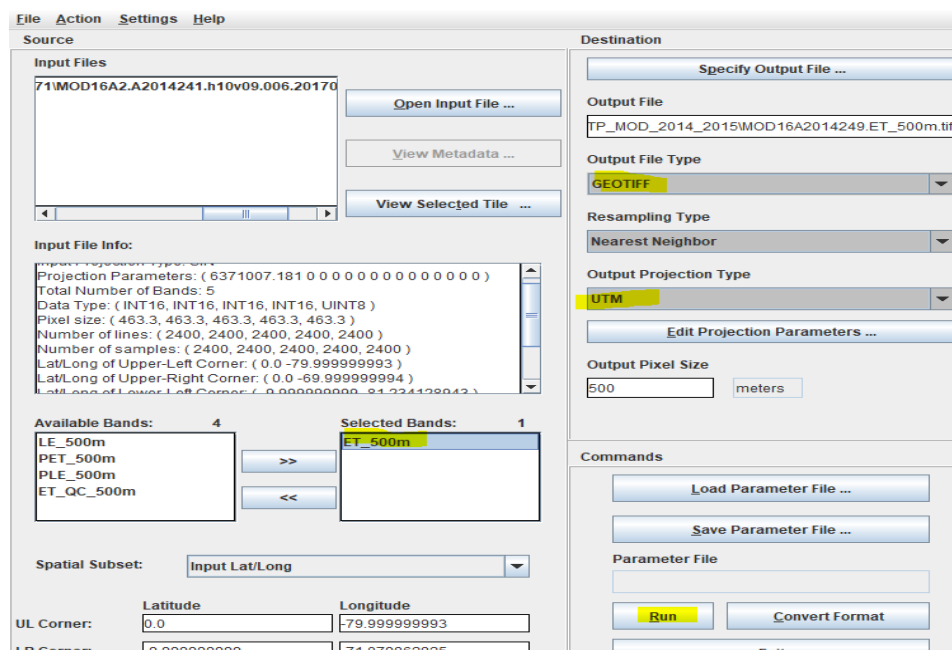
Figura 25. Selección, proyección y cambio de formato de las imágenes MODIS
