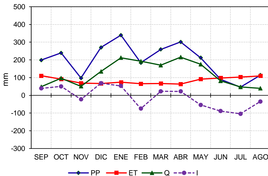
Figura 17. Acumuladas mensuales para el área de captación de la cuenca Challana. Precipitación (P), evapotranspiración real (ETr), Gasto de agua (Q) y la diferencia (P-(ETr+Q)) de un año de análisis septiembre 2014 - agosto 2015.
