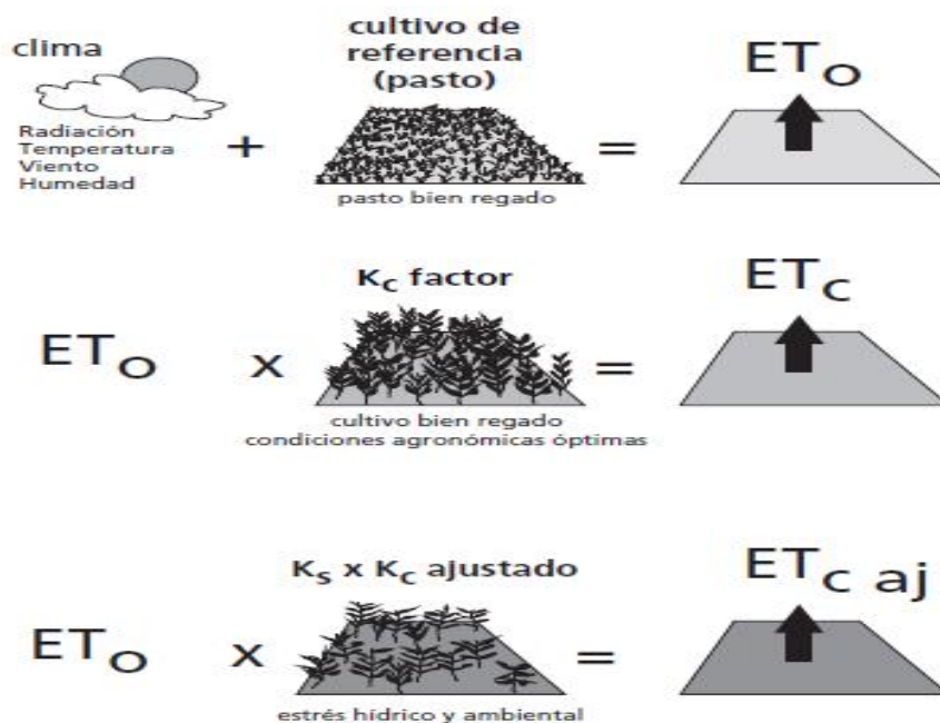
Figura 3. Evapotranspiración del cultivo de referencia ( ET_0 ), bajo condiciones estándar ( ET_c ) y bajo condiciones no estándar ( ET_{c\ aj} ). Fuente: ALLEN et al , 2006
