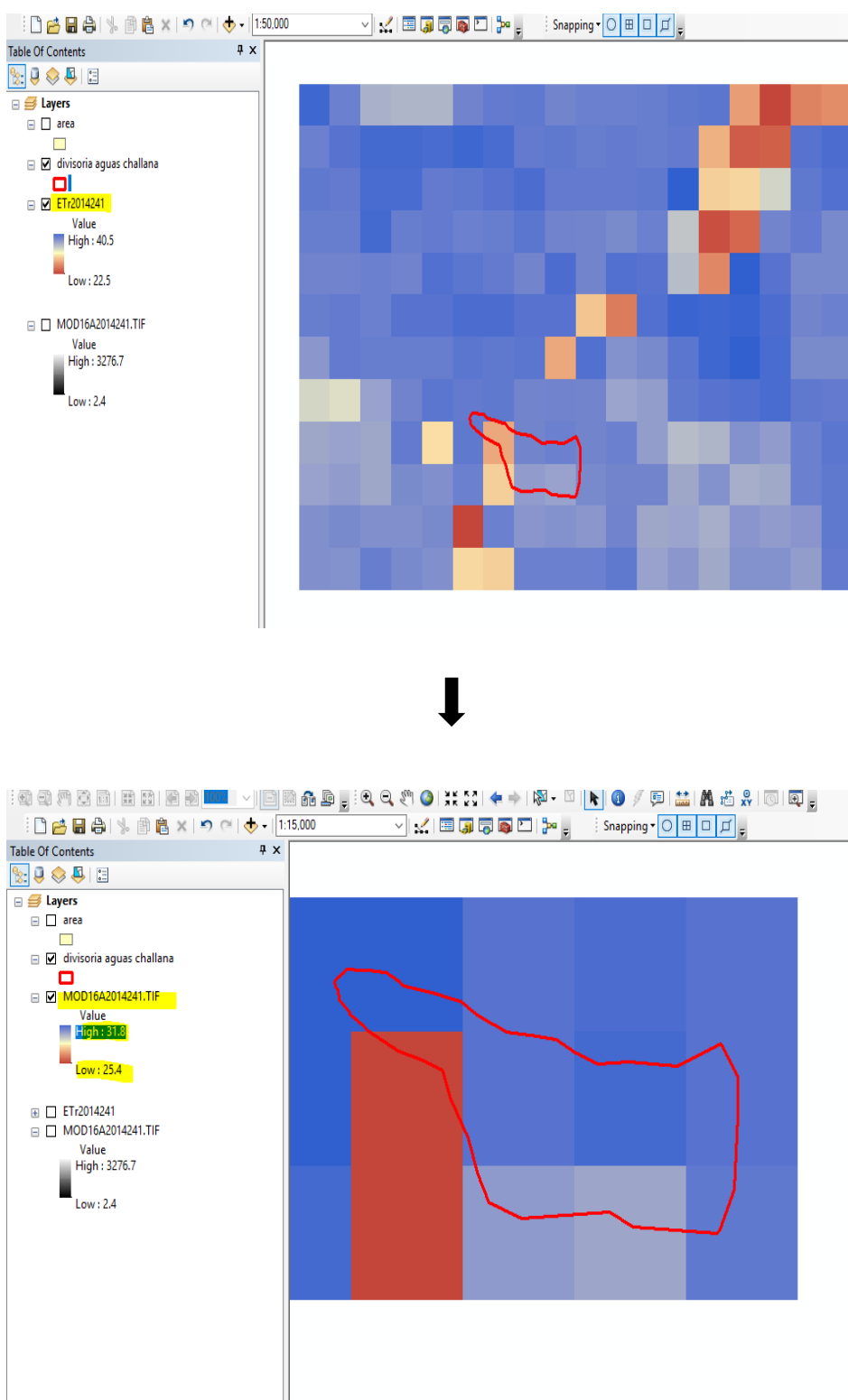
Figura 28. Extracción de área de interés de un tamaño de pixel de 3 x 5
